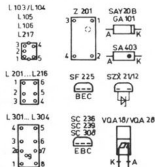
Spulen, Filter, Halbleiterbauelemente auf die Anschlüsse gesehen
