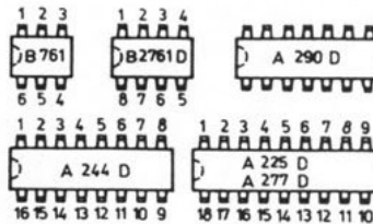
Schaltkreise auf die Anschlüsse gesehen
