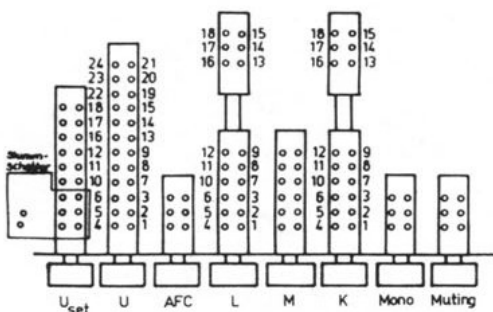
Schiebetastenschalter von oben gesehen
